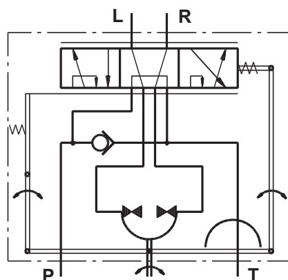
"Отворен център – с реакция" HKU.../3
