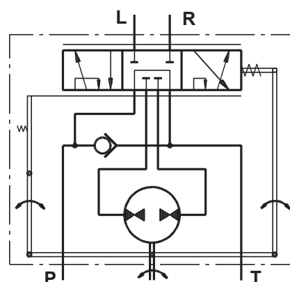
"Отворен център – без реакция" HKU.../4
